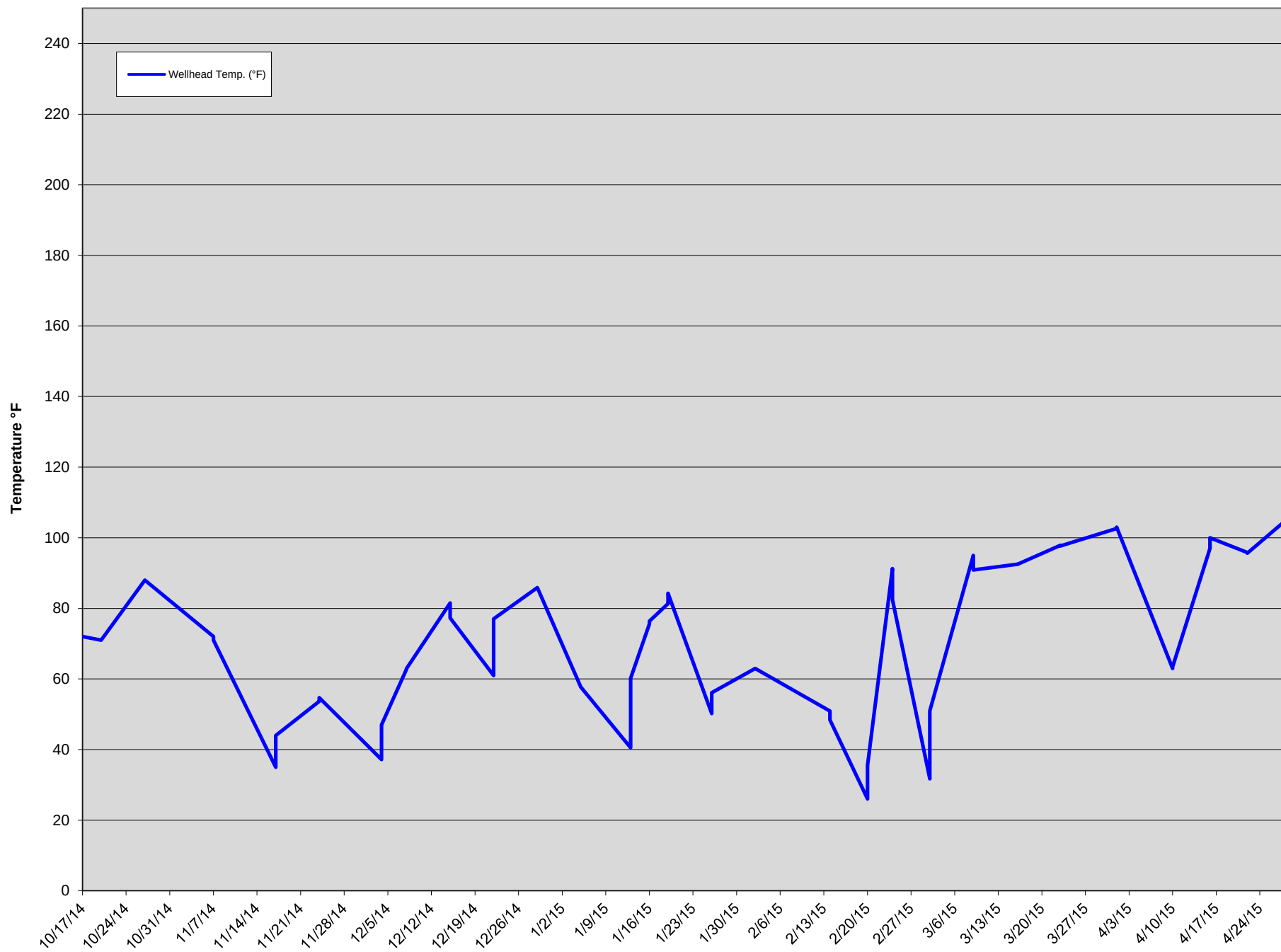
GEW-010 Wellhead Temperatures
